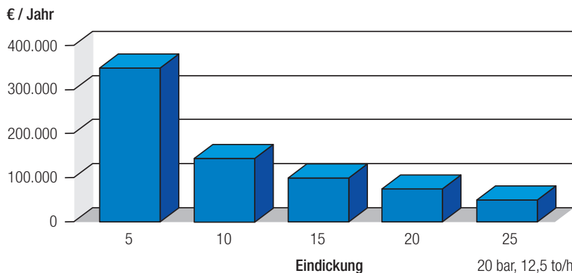
Energieverluste reduzieren durch Anhebung der Eindickungszahl.
